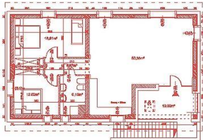
PIĘTRO
