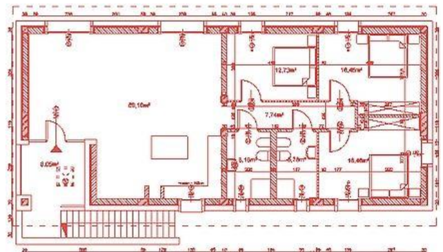
PIĘTRO
