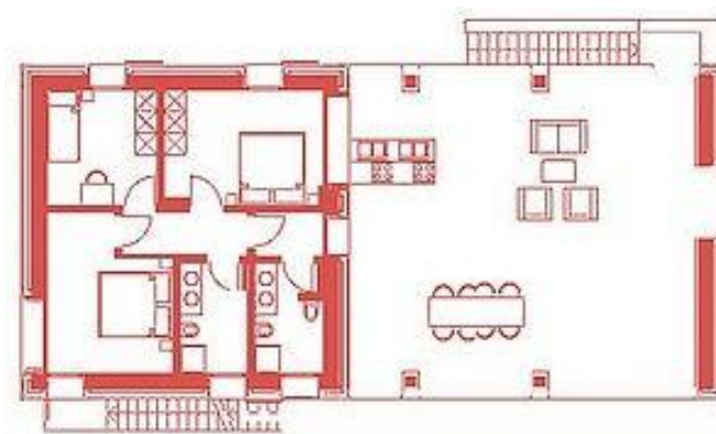
PIĘTRO
