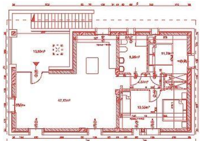
PIĘTRO
