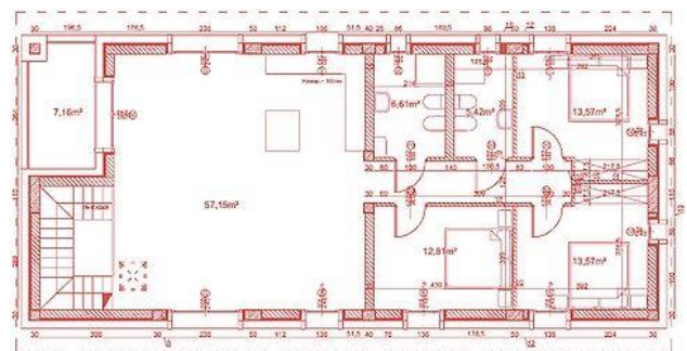
PIĘTRO
